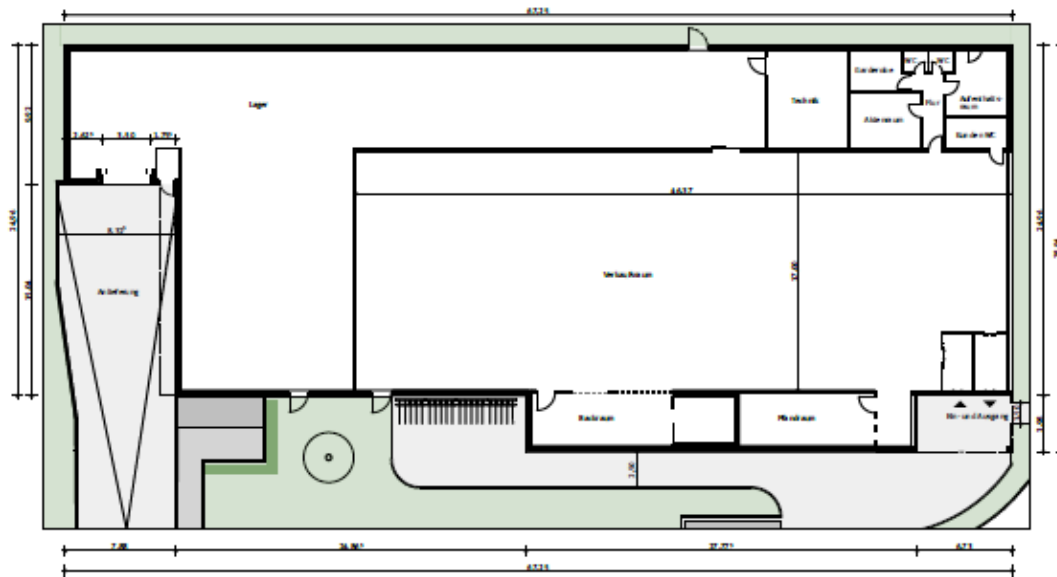
Grundriss Lebensmittel-Discountmarkt
